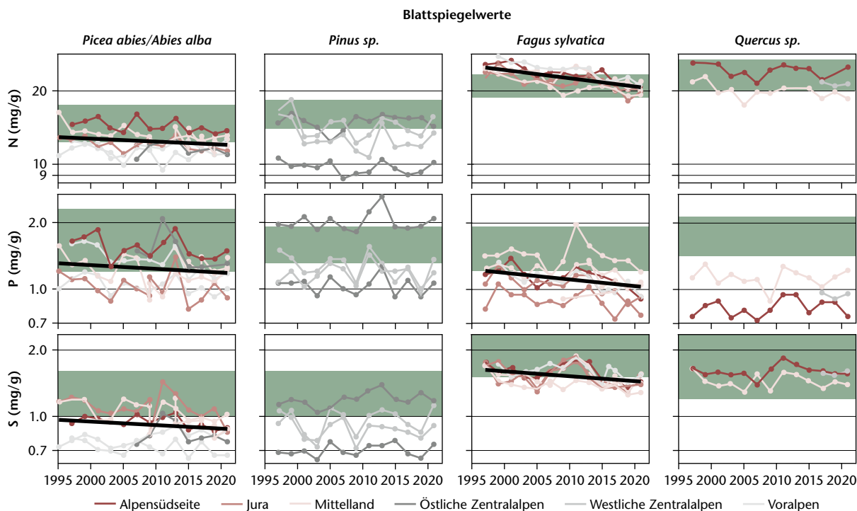
Abb 6 Zeitliche Trends der Konzentration von Stickstoff (N), Phosphor (P) und Schwefel (S) in den diesjährigen Blättern von vier Baumartengruppen. Schattierte Bereiche kennzeichnen den Normalbereich der Nährstoffkonzentrationen nach Mellert & Göttlein (2012). Schwarze Trendlinien zeigen signifikante Trends.
